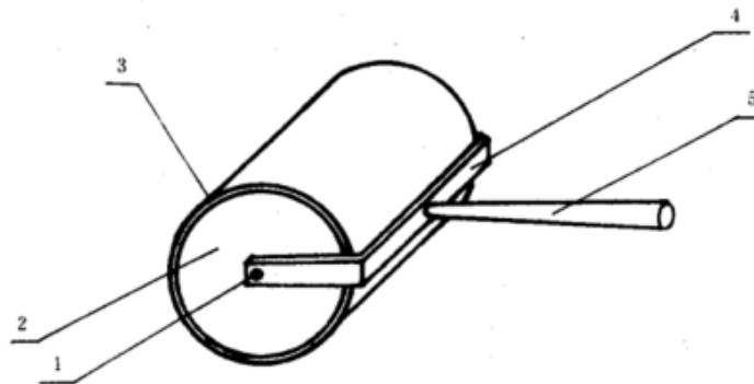
图5 滚筒示意图
